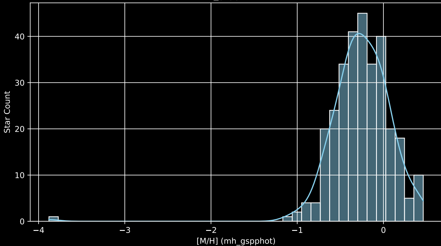
GALAH DR4 Field: [465] [M/H] (mh_gspphot) (n= 303)
