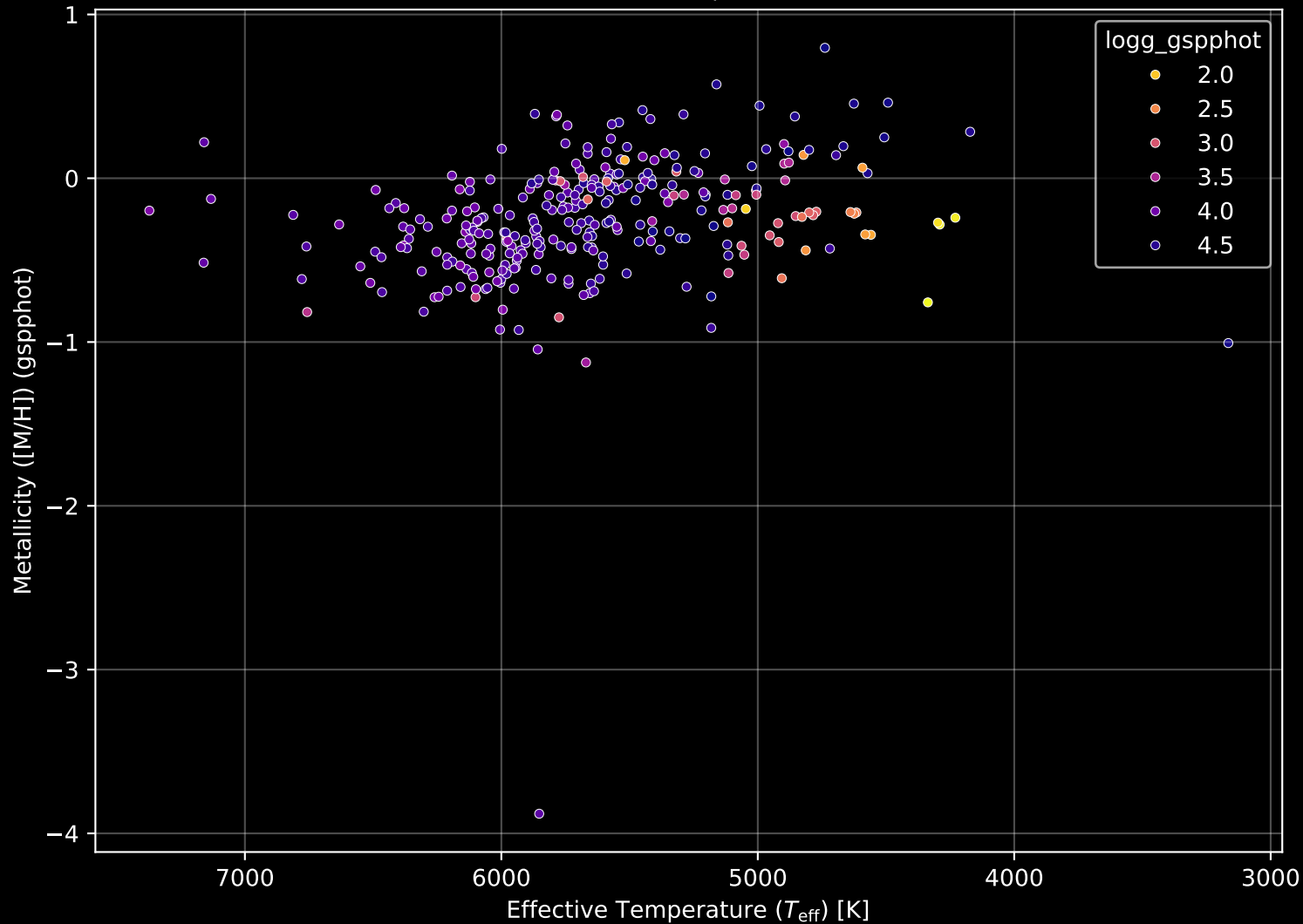
GALAH DR4 Field: [465] Stellar Population Parameters (n= 305)
